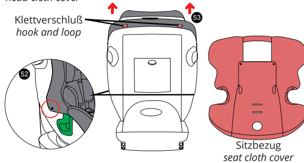
Schrittpolster crotch pad
